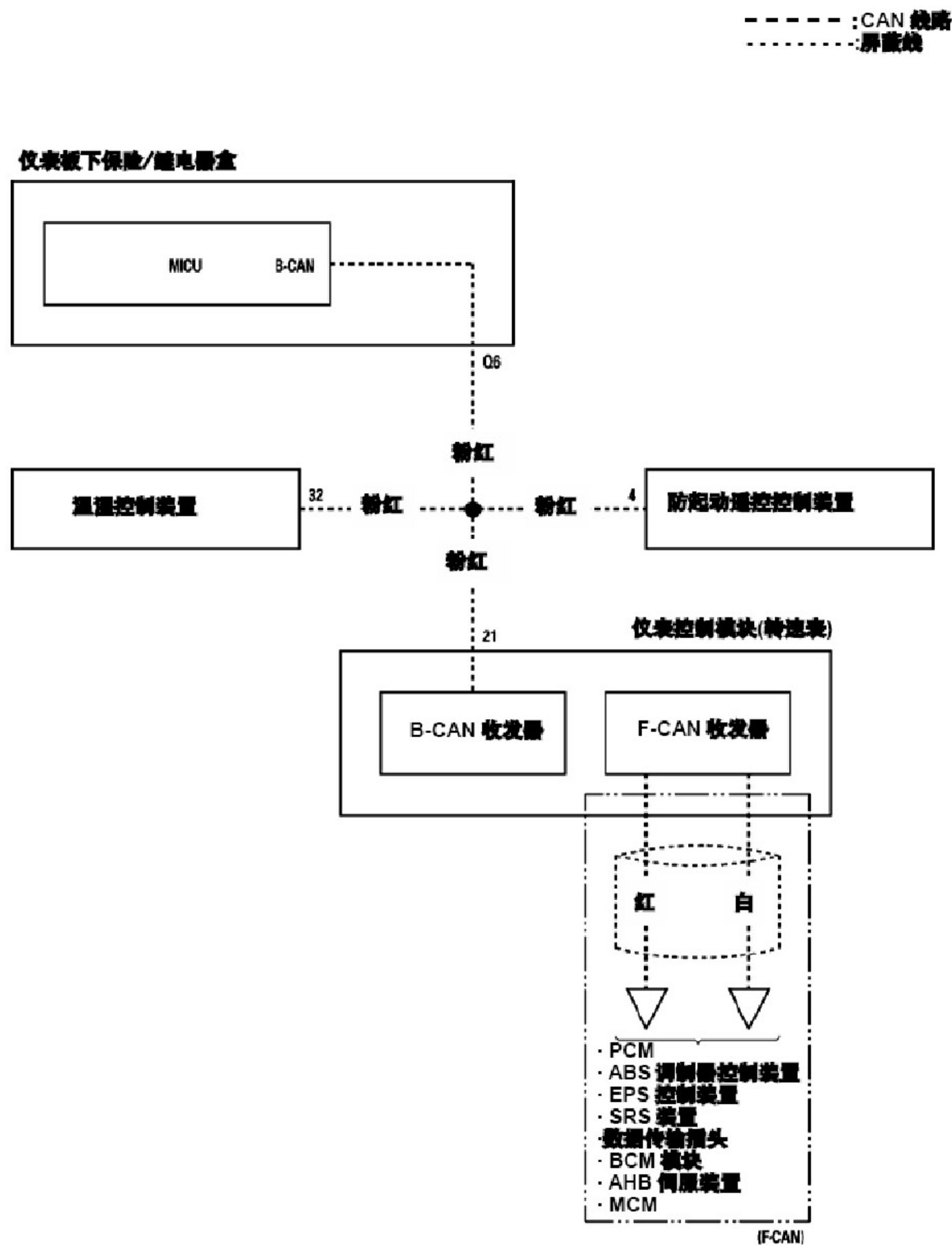
电路图
