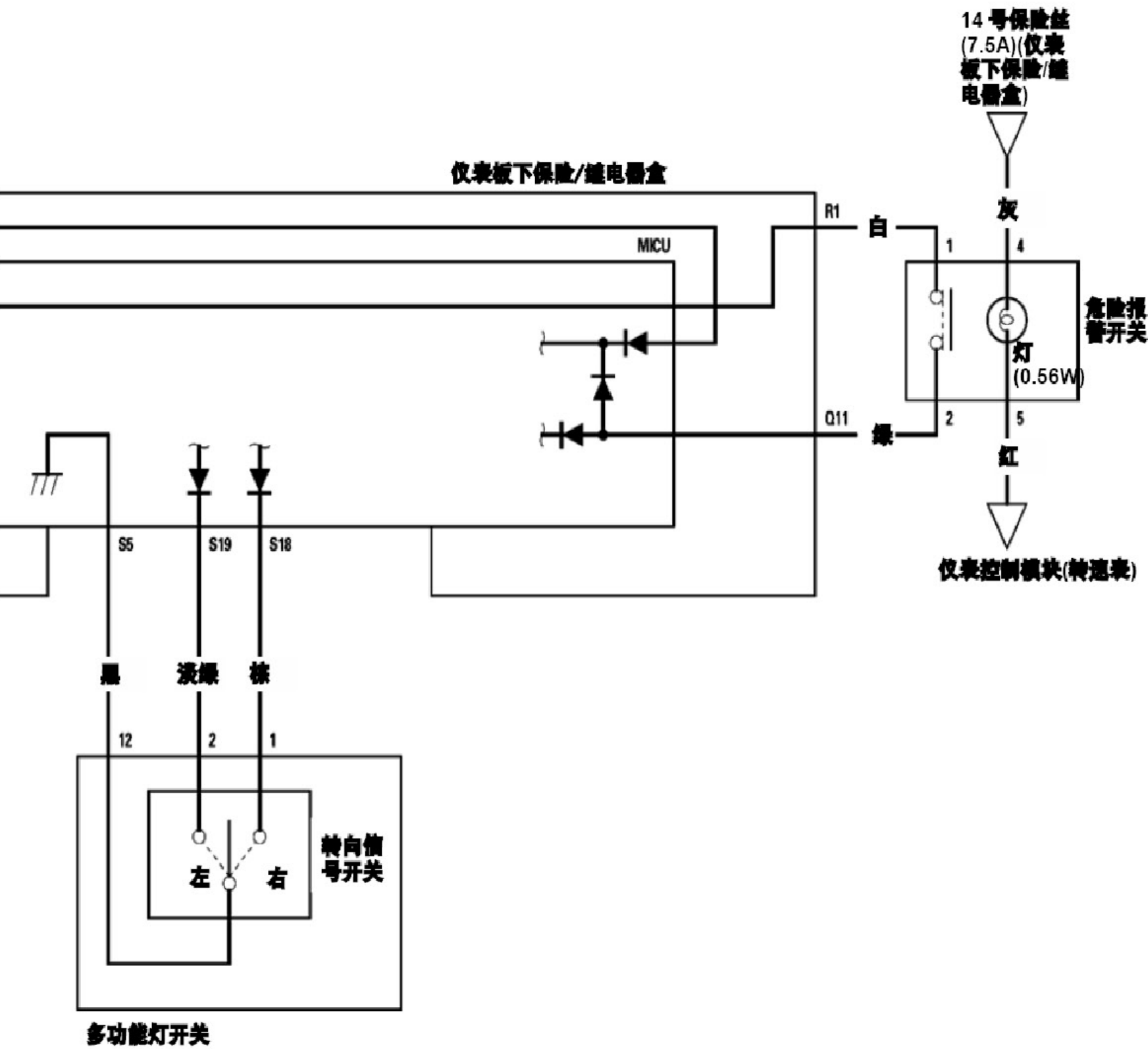
电路图（续）
