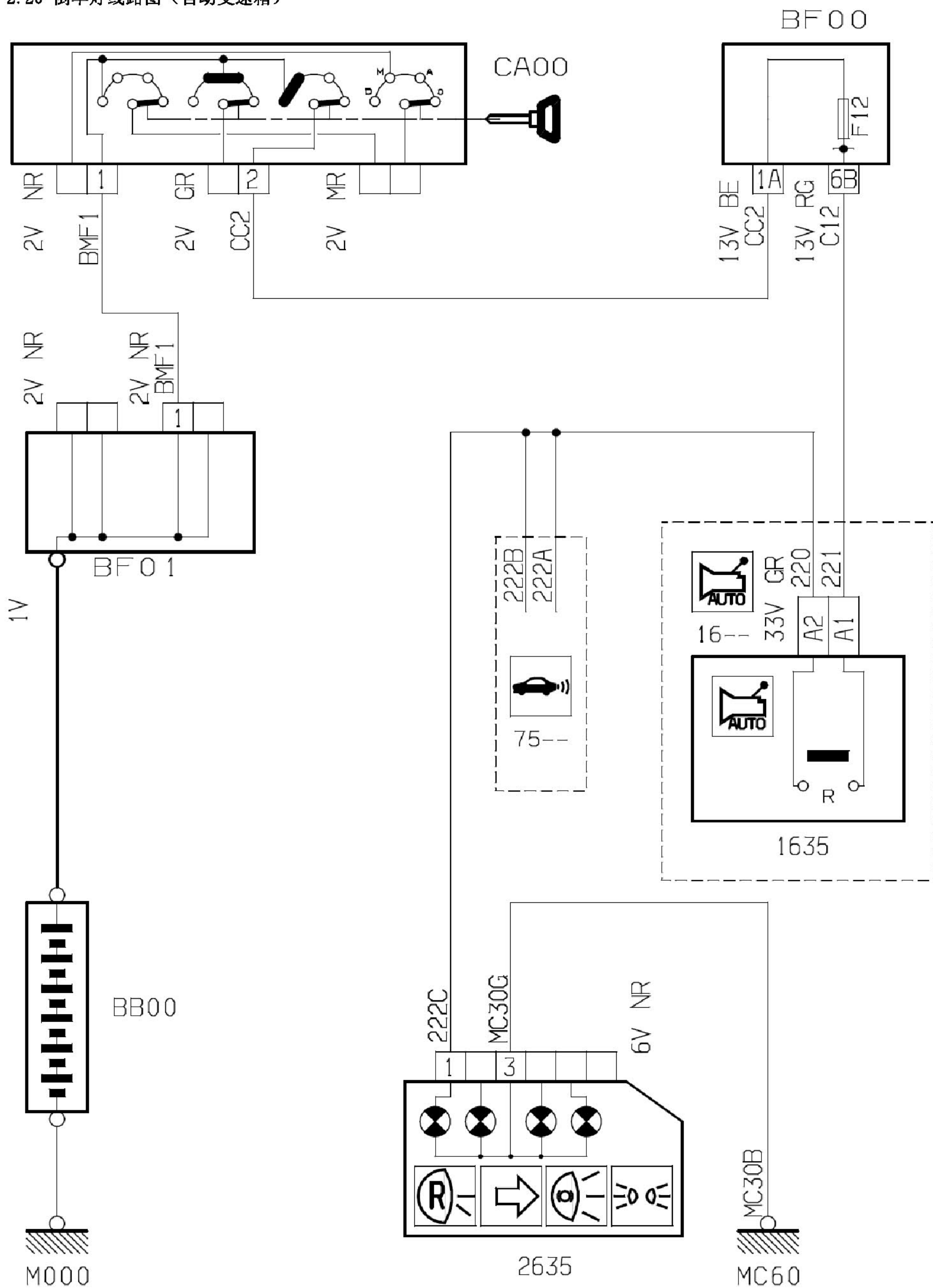
2.20 倒车灯线路图（自动变速箱）
